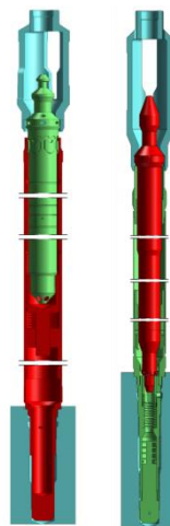
控制棒换料专用套筒和抓具
